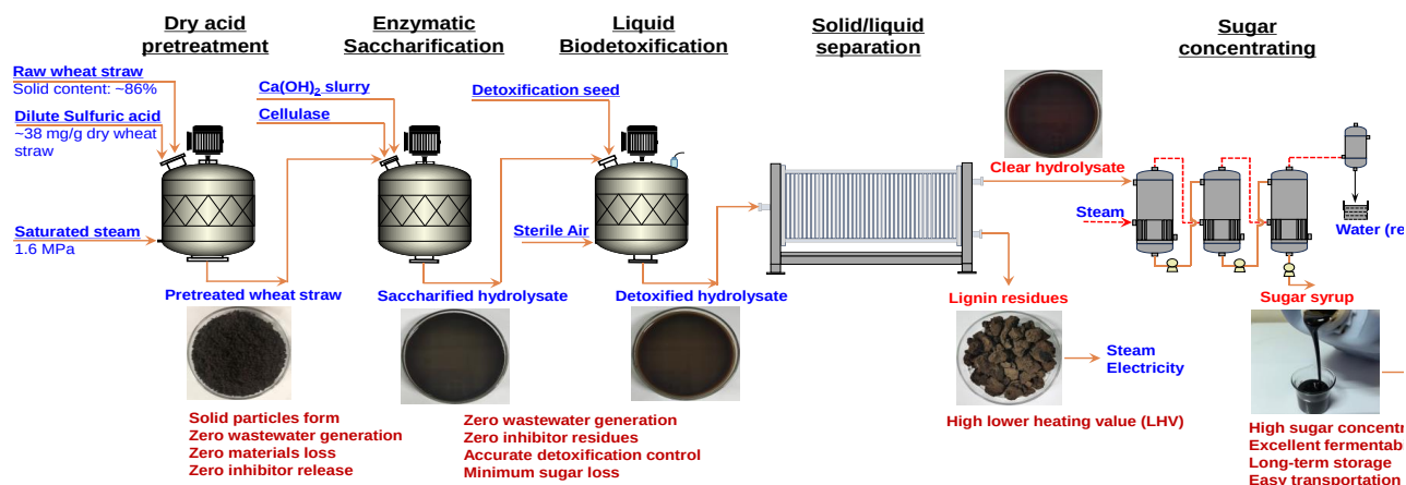
图1 干法生物炼制生产秸秆糖及其升级转化示意图
